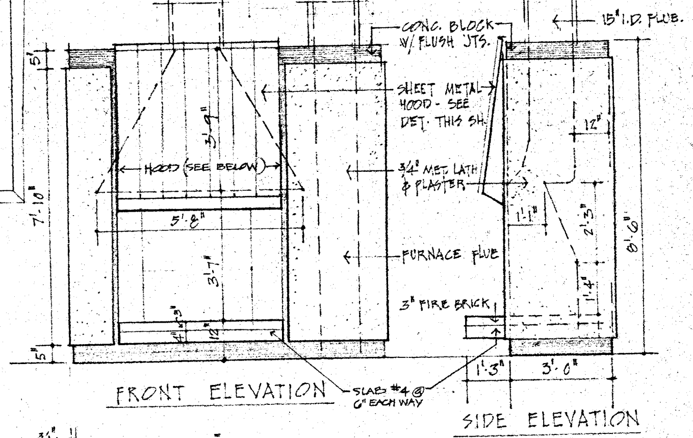
FIREPLACE DETAILS SCALE: 3/8" = 1'-0"
